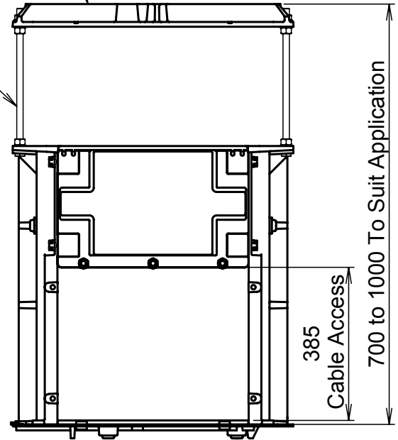
End Elevation
