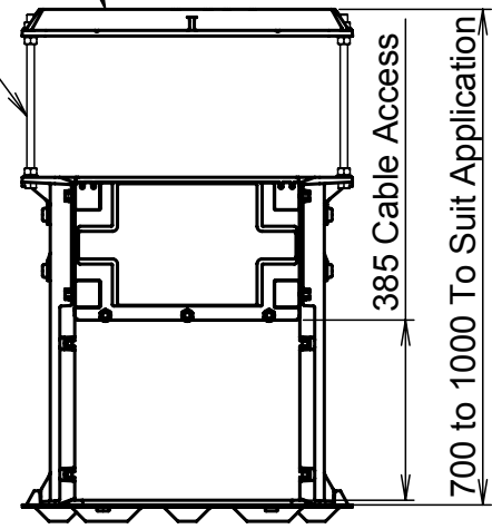
End Elevation
