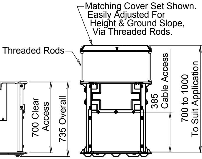
End Elevation
