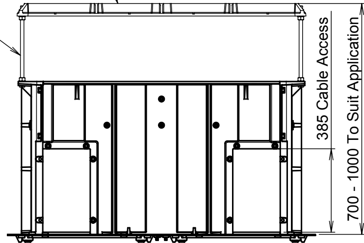
End Elevation
