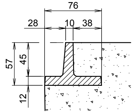
Section A-A Typ Frame
