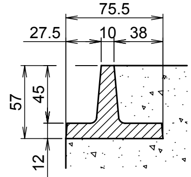
Section A-A Typ Frame
