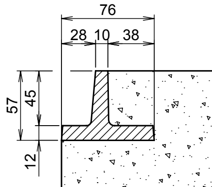
Section A-A Typ Frame
